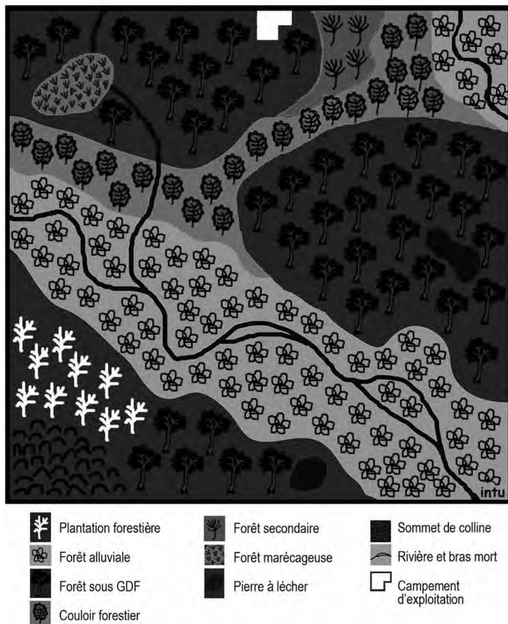
Figure 4. Représentation schématique d'un paysage forestier
